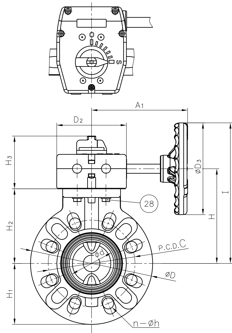
DIMENSIONS TABLE
