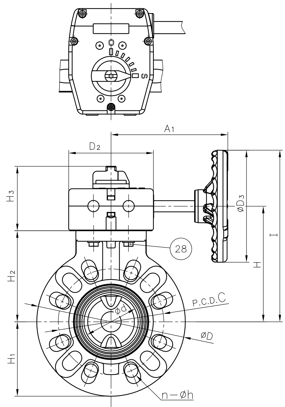
DIMENSIONS TABLE
