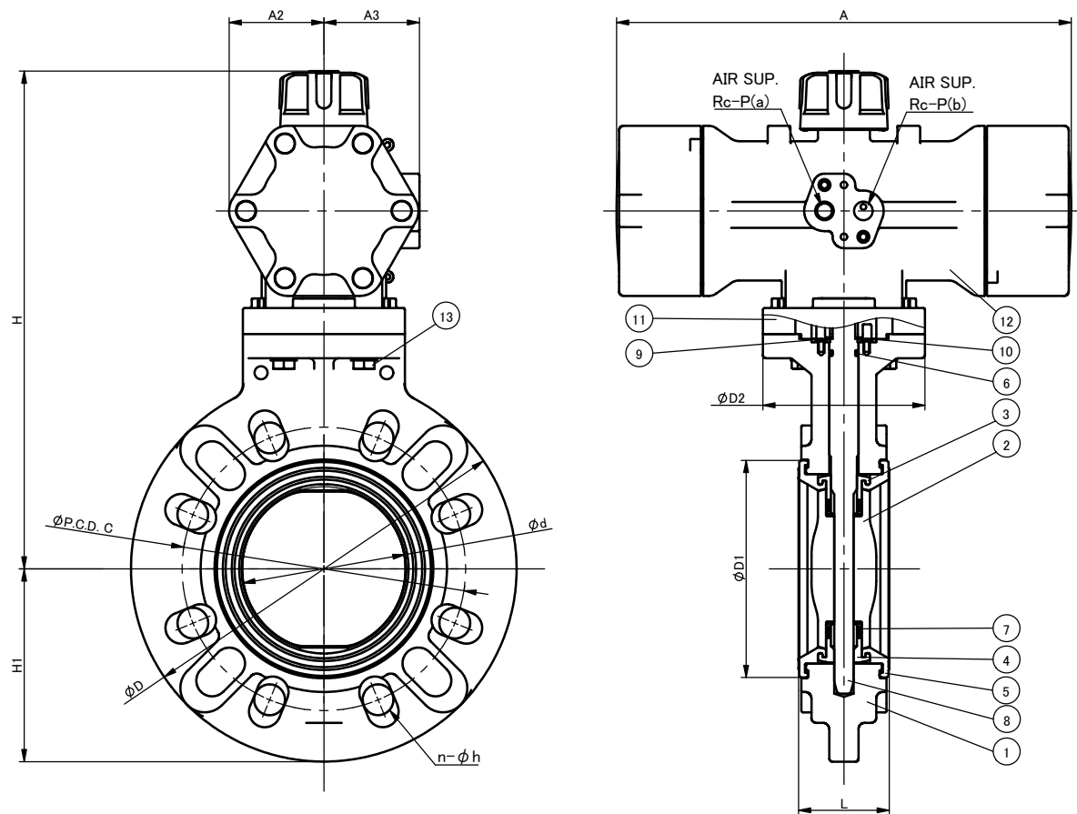
DIMENSIONS TABLE
