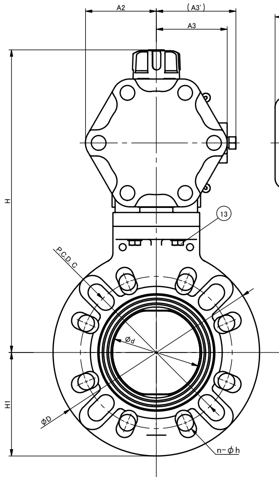
DIMENSIONS TABLE
