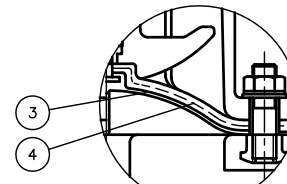
PTFE diaphragm.
