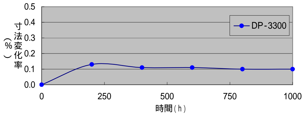
高湿下の寸法変化率(65%、90%)
