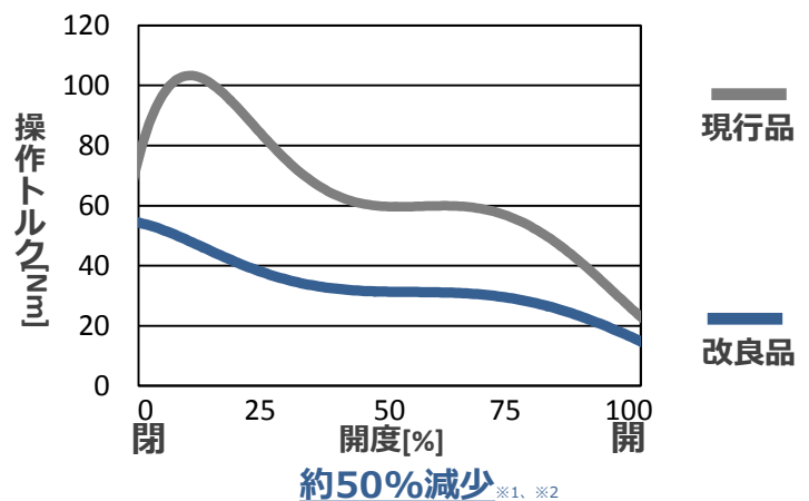
開度毎の操作トルク:300mm (閉→開)
