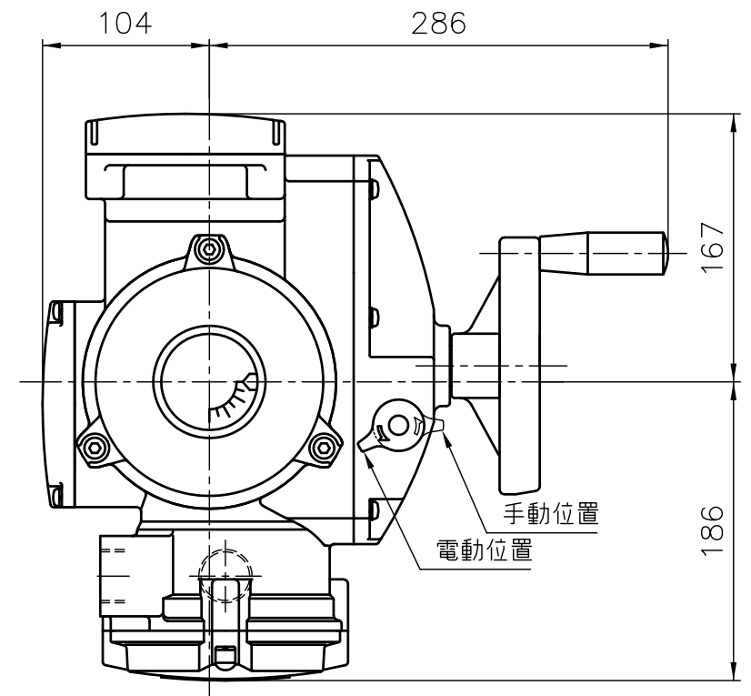
X-X 矢視図
