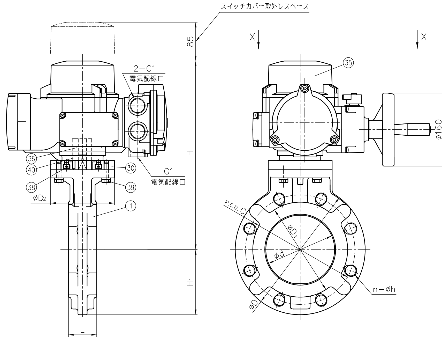
寸法表
