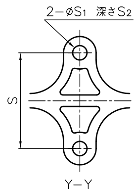
(エンザート金具取付穴部詳細)
