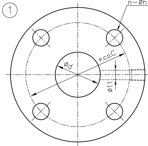
DIMENSIONS TABLE
