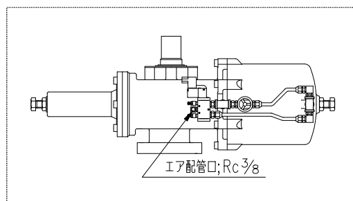
(図 2)電磁弁・フィルタ付減圧弁付
