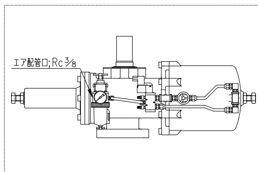
(図 2)電磁弁・フィルタ付減圧弁付
