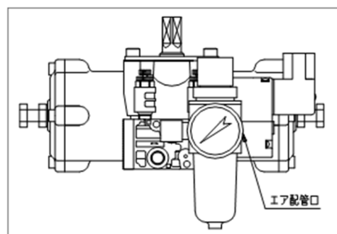
(図 2)TA 型 電磁弁・フィルタ付減圧弁
