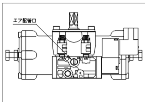
(図 1)TA 型 電磁弁付
