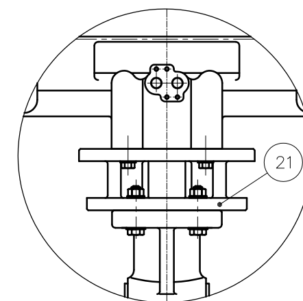
呼び径200mm,250mm用取付台形状
