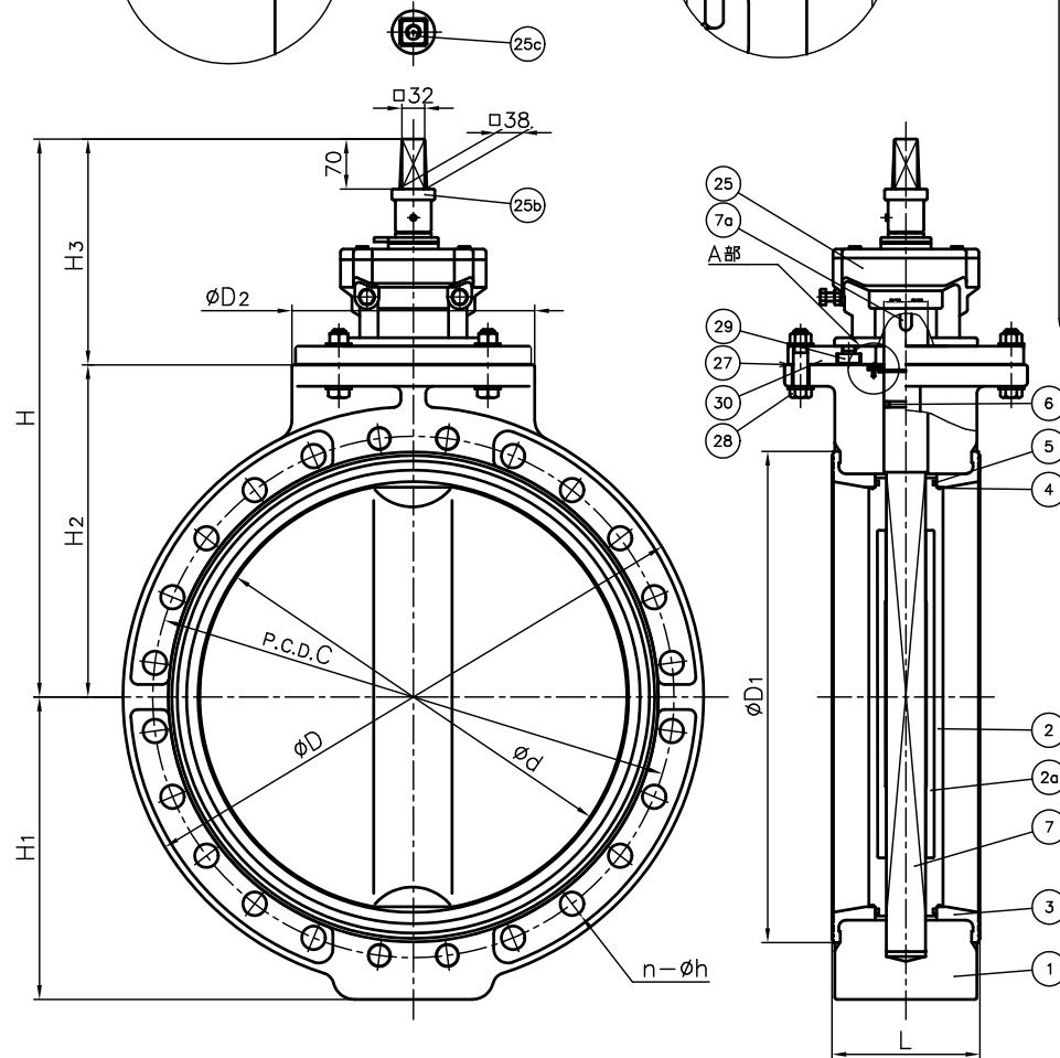
寸法表
