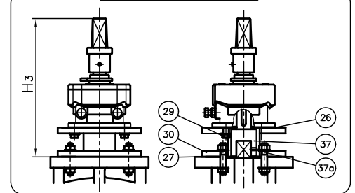
400mm取付台・駆動部
