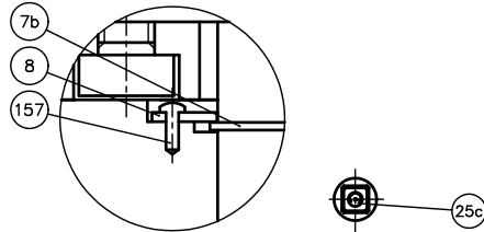
A部詳細図 (450~600mmの場合)
