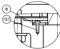
A部詳細図 (400mmの場合)
