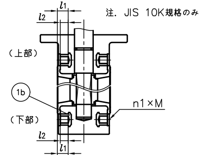
ボディ埋込金具詳細
