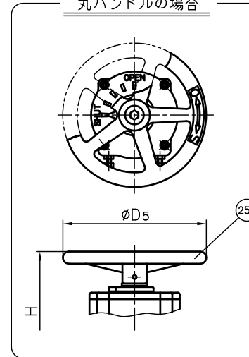
丸ハンドルの場合
