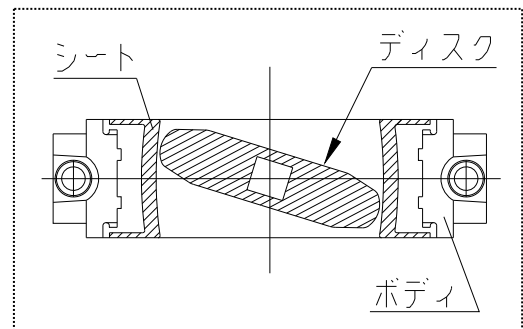
参考図
