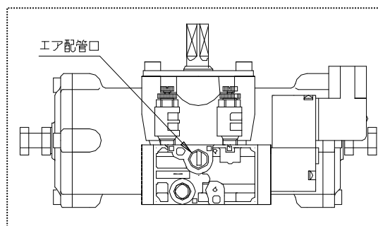
(図 1)電磁弁付
