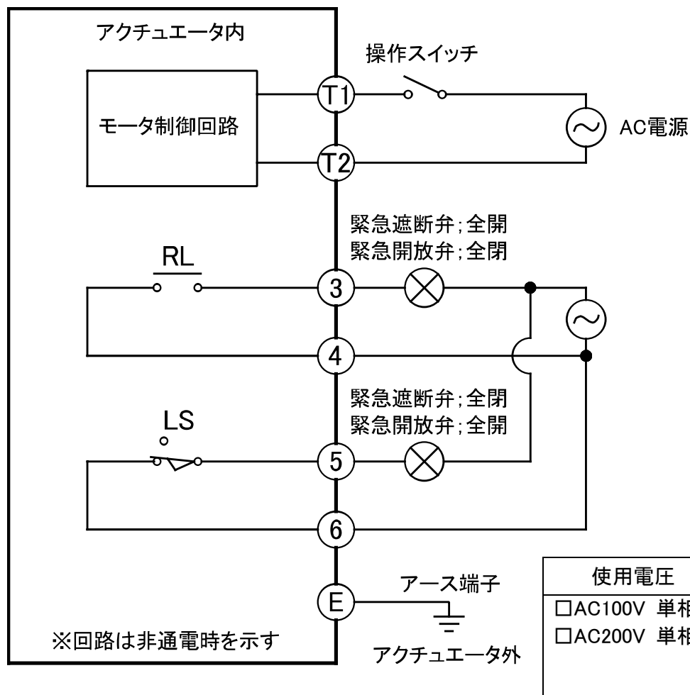
スイッチングチャート (2 線式)
