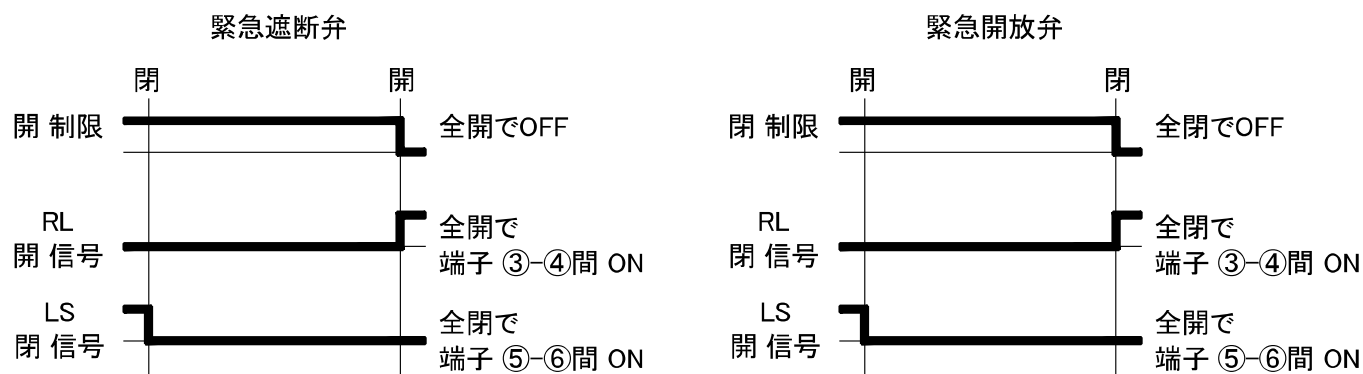
スイッチングチャート (2 線式)
