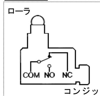
内部回路図
