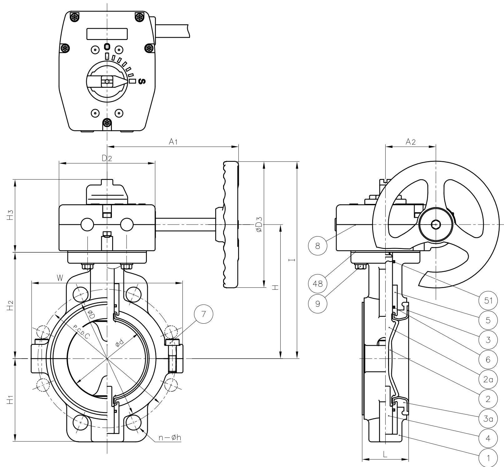
寸法表
