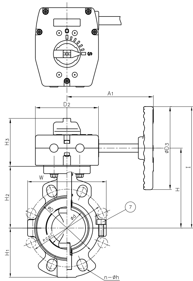
寸法表
