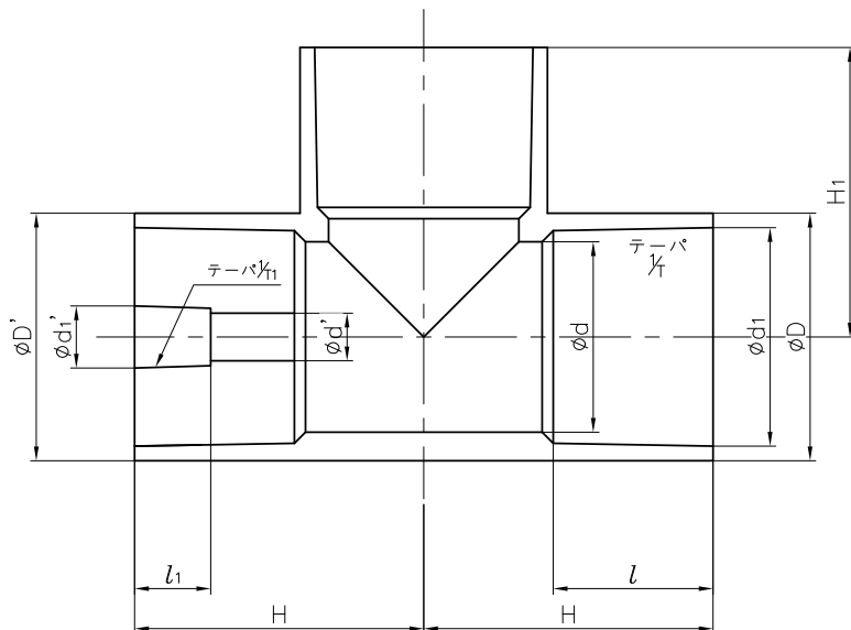
接着タイプ
