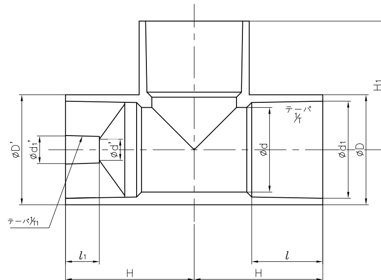
溶着タイプ
