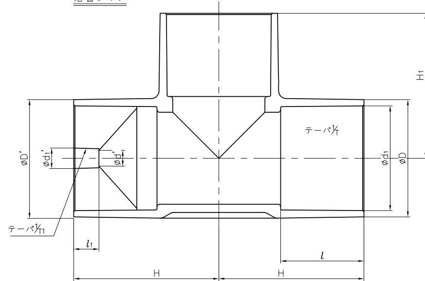
溶着タイプ
