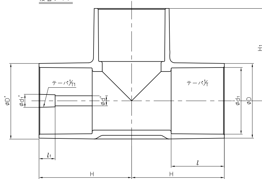
接着タイプ
