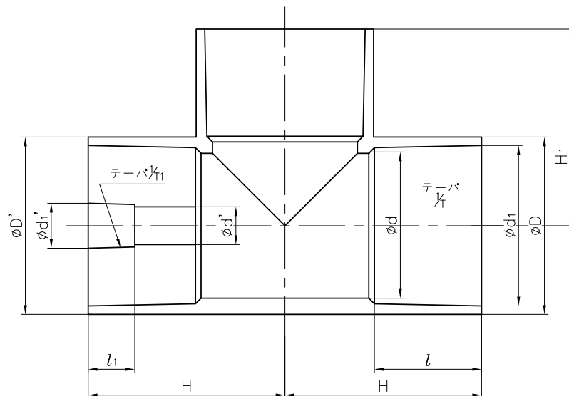
接着タイプ
