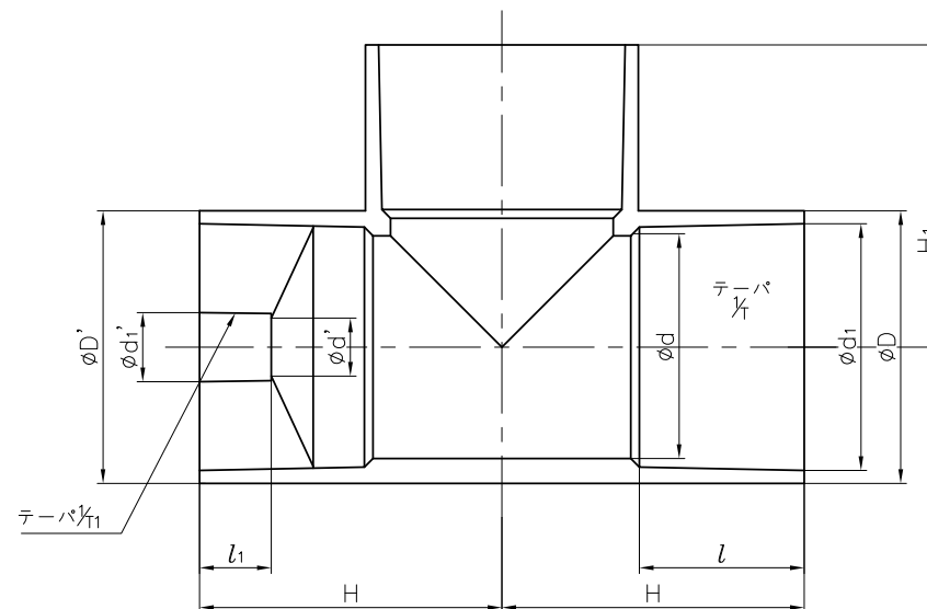
溶着タイプ
