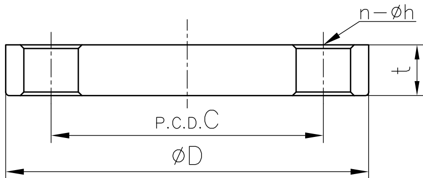
寸法表
