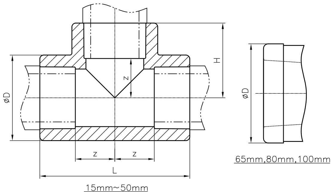
寸法表
