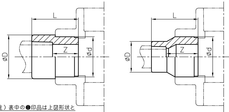
寸法表
