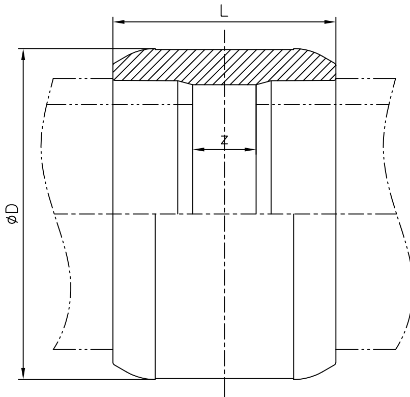
寸法表
