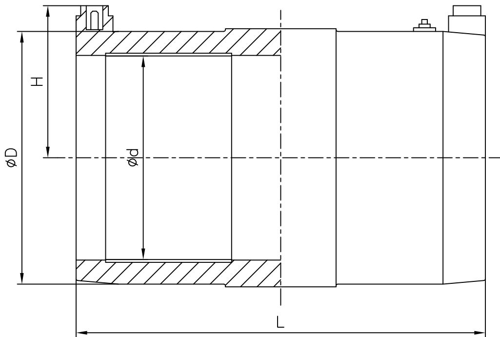
寸法表
