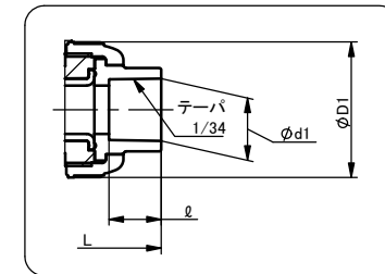
ソケット形
