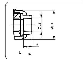
ねじ込み形
