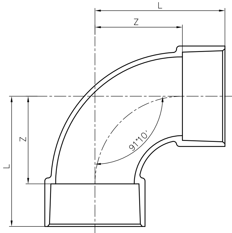
寸法表
