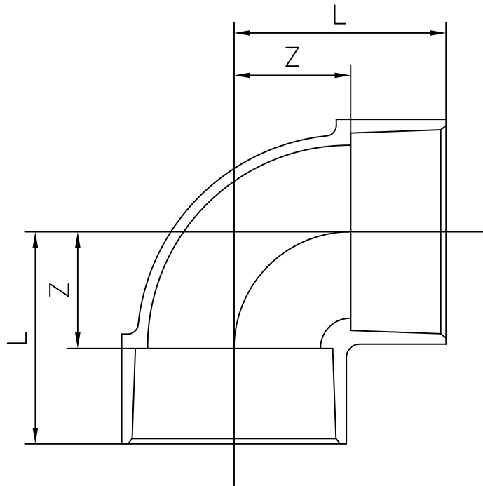
寸法表 単位 : mm
